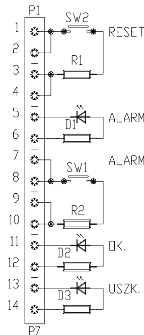
Rys. 19 Schemat elektryczny przycisku RPO-1a
