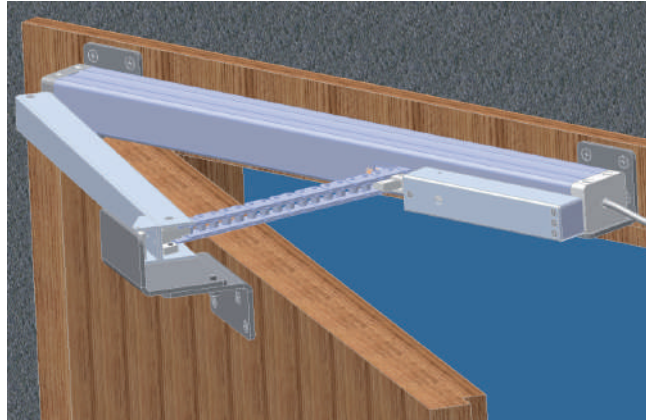
Rys. 51 Otwieranie do wewnątrz
