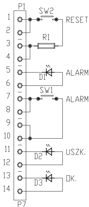
Rys. 18 Schemat elektryczny przycisku RPO-1
